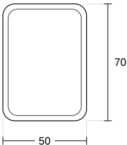
DALL'ALTO
